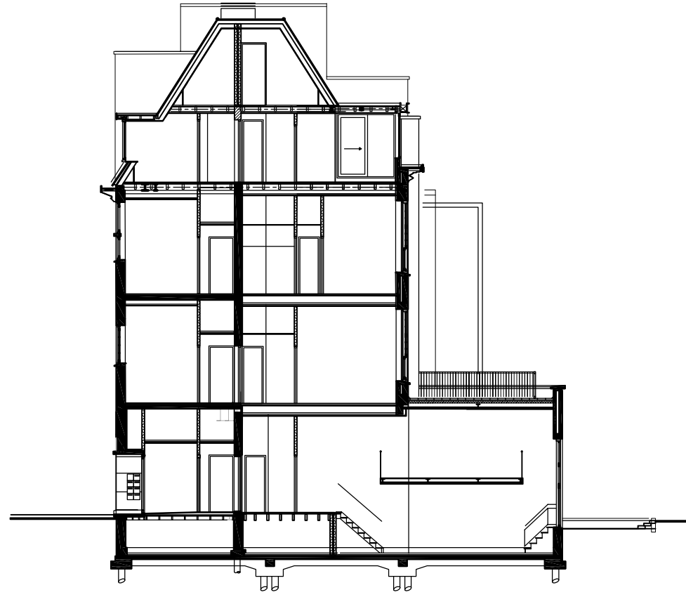
doorsnede B-B
