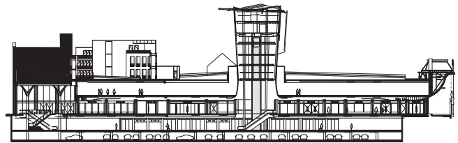
doorsnede
