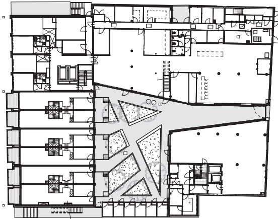
begane grond
