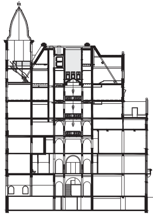
doorsnede
