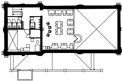
eerste verdieping
