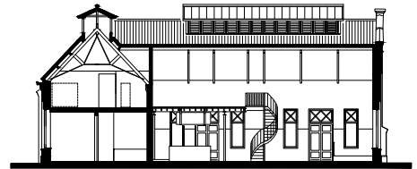
langsdoorsnede
