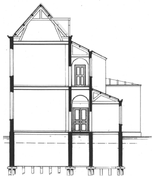
doorsnede
