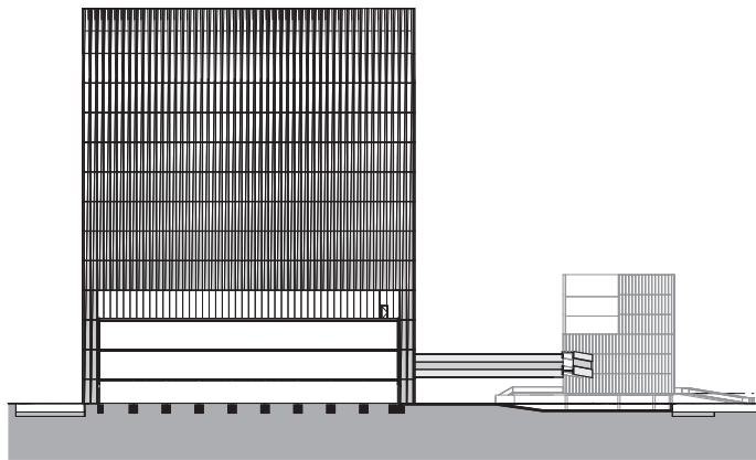
voorgevel
