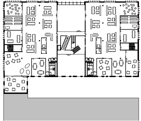
eerste verdieping
