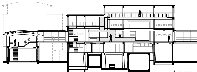
doorsnede
