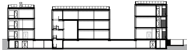
langsdoorsnede
