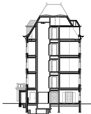
dwarsdoorsnede
