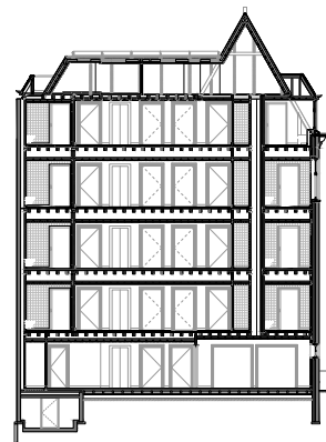
langsdoorsnede
