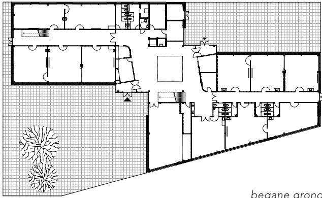
begane grond
