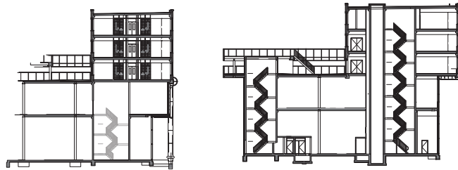
langsdoorsnede
