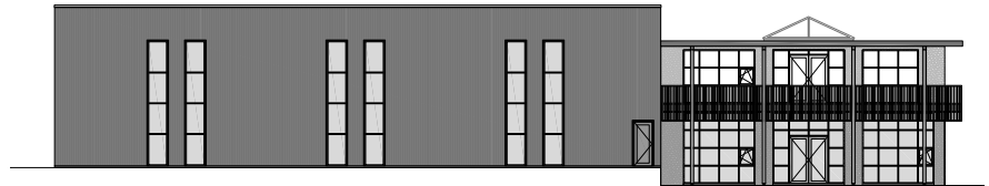
noordwestgevel
