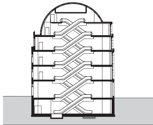
doorsnede
