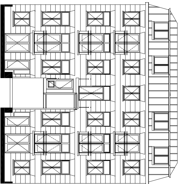
Achtergevel
