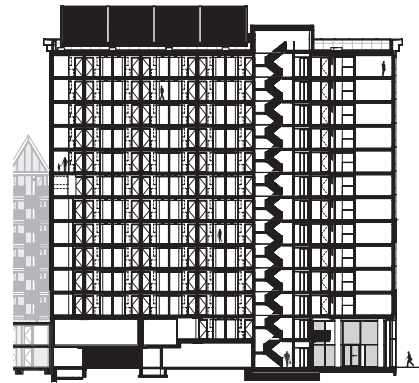
doorsnede
