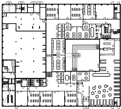
begane grond
