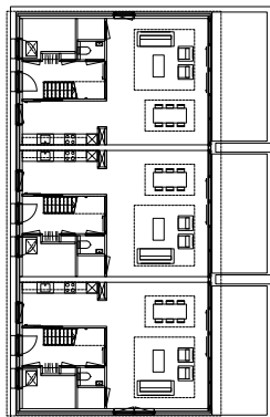
begane grond
