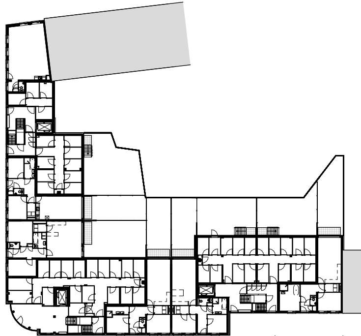
begane grond
