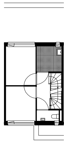
1e verdieping
