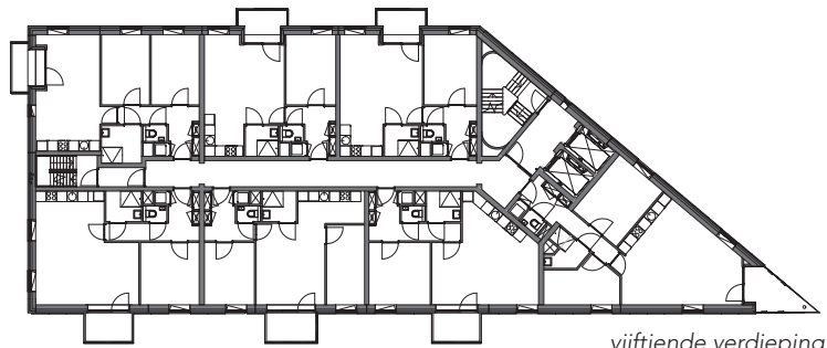
vijftiende verdieping
