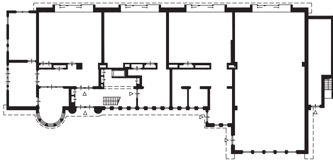
begane grond
