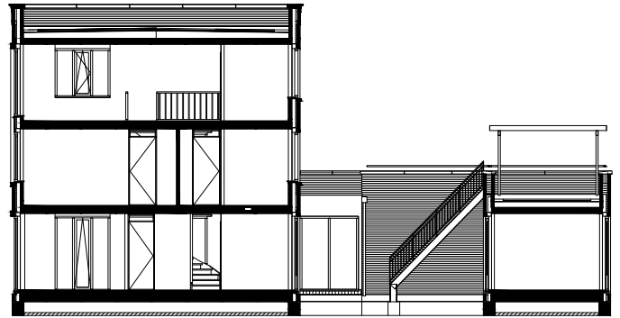
doorsnede
