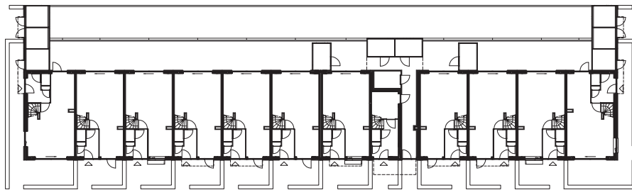
begane grond blok 1.3
