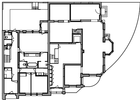
begane grond
