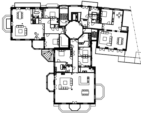
eerste verdieping
