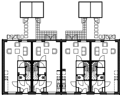
begane grond
