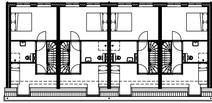
eerste verdieping
