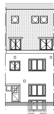
voorgevel
