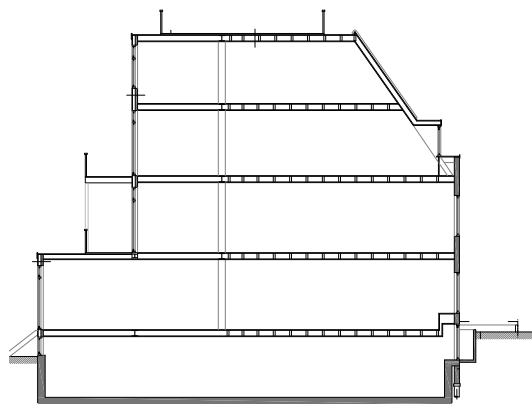
dwarsdoorsnede
