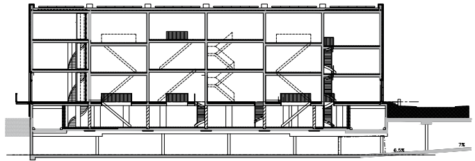
doorsnede
