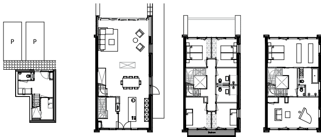
souterrain, begane grond, eerste en tweede verdieping
