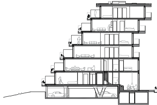
dwarsdoorsnede
