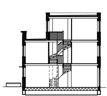
doorsnede
