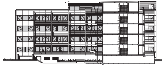
doorsnede
