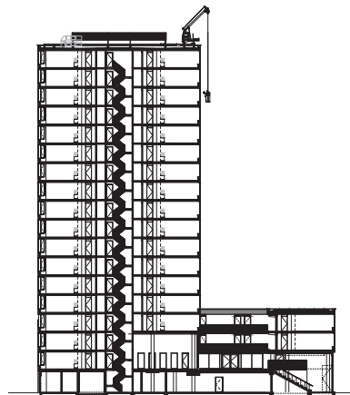
doorsnede
