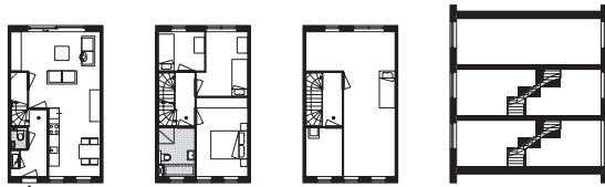
rijwoning
