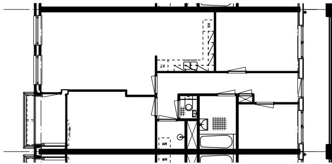
WONINGTYPE C1 1e verd
