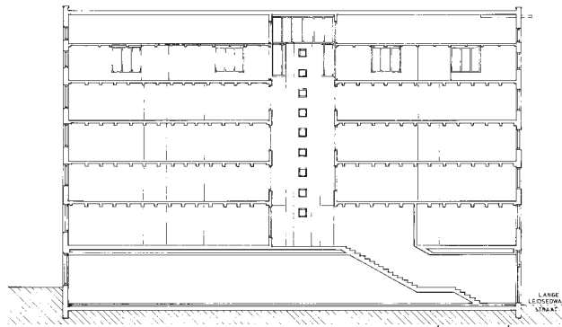
doorsnede
