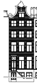
voorgevel
