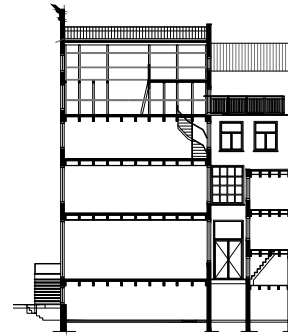
doorsnede
