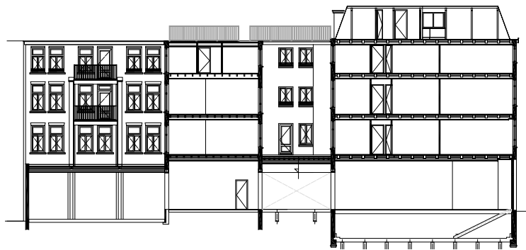
doorsnede
