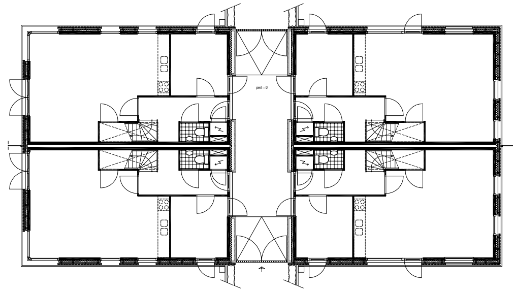
BEGANE GROND
