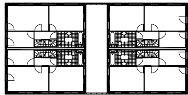
EERSTE VERDIEPING
