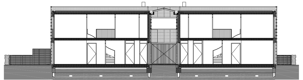
DOORSNEDE huurwoning
