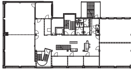
vierde verdieping
