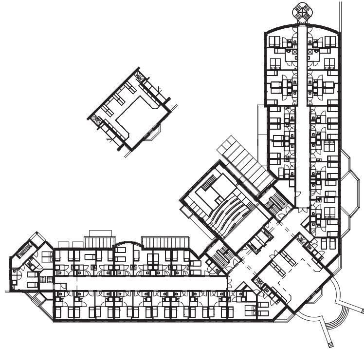
eerste verdieping
