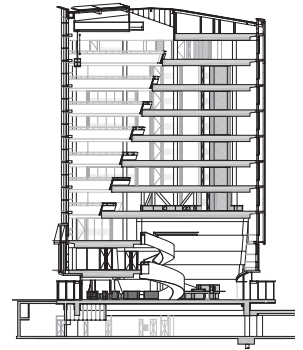
doorsnede
