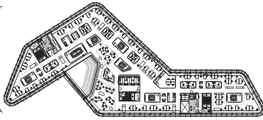
zesde verdieping
