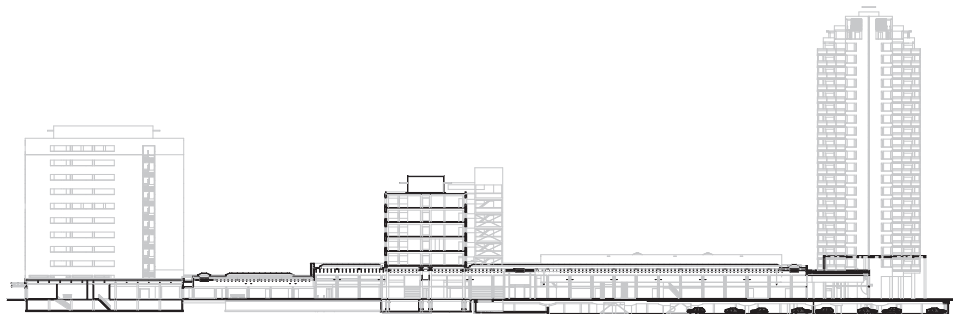
doorsnede
