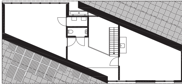
begane grond
