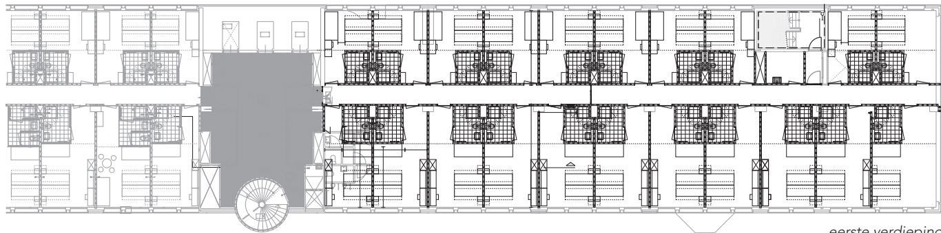
eerste verdieping
