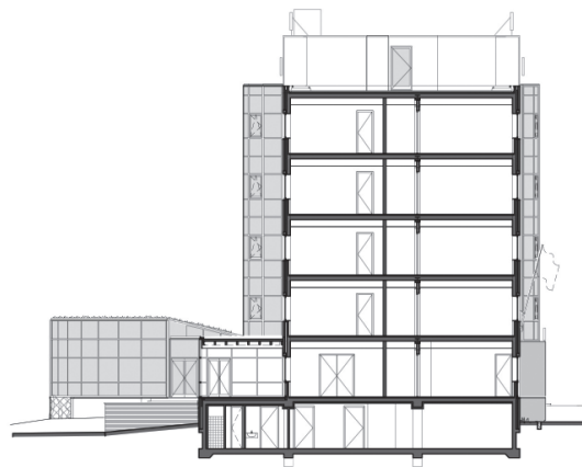
doorsnede
