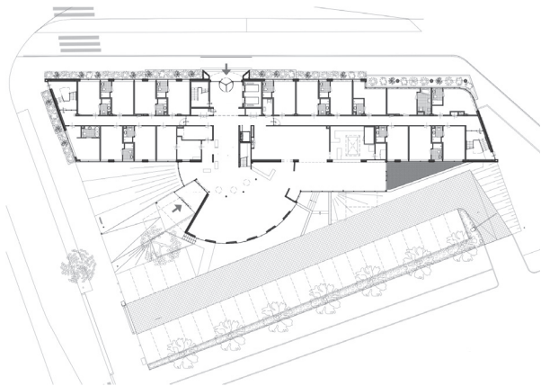
situatie en begane grond
