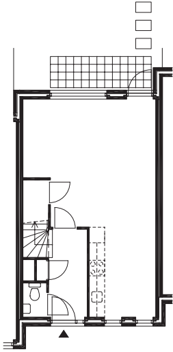
begane grond
