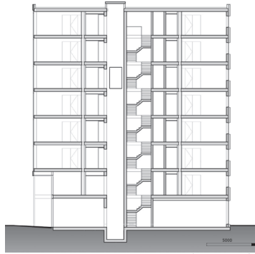
doorsnede
