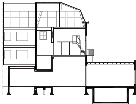
doorsnede
